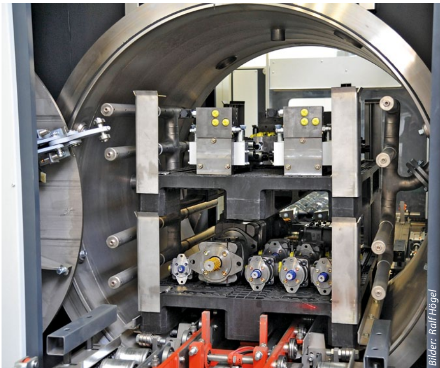
Das maximale Chargengewicht bei doppelstöckiger Beladung der Arbeitskammer beträgt 1000 Kilogramm
